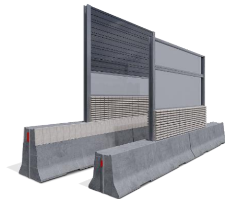
DB NBF-serien är en del av det passiva helhetskonceptet DELTABLOC® har tagit fram. Att integrera en bullerskyddsvägg i skyddsbarriärsystemet sätter en ny teknisk standard för trafiksäkerhet och bullerskydd. Vid användning av bilden vänligen ange: © KIRCHDORFER Road & Traffic
